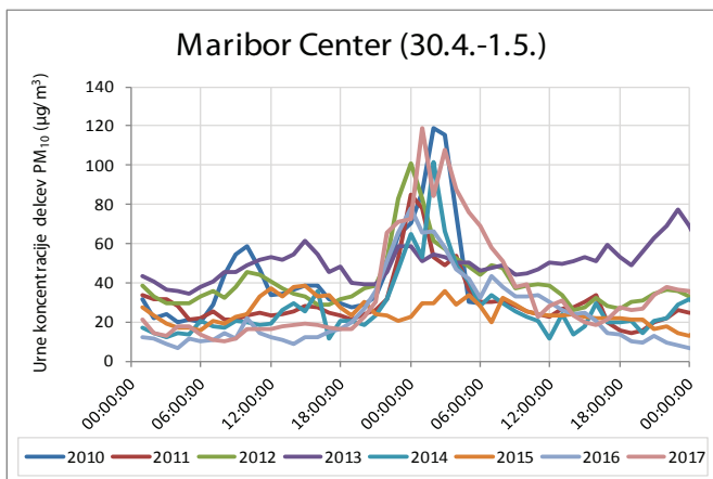
Vpliv kurjenja na koncentracije delcev PM10 se vidi kot poviševanje izmerjenih vrednosti na dan 30. 4. kmalu po 20:00, ki dosežene najvišje koncentracije na dan 1. 5. od polnoči do 03:00
