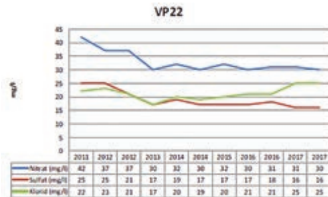
Vsebnost nitrata, sulfata in klorida (mg/l) v podzemni vodi na opazovalni vrtini VP 22 v letih 2011–2017
