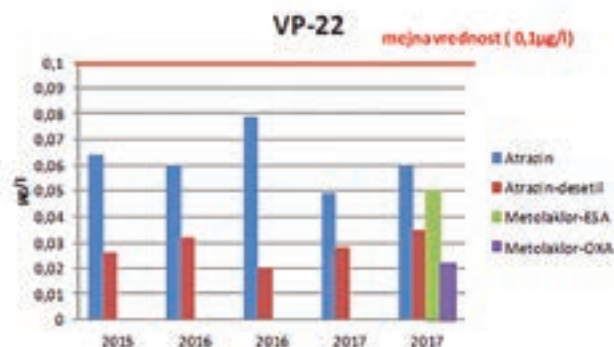
Vsebnost atrazina, desetil-atrazina ter metolaklora ESA (µg/l) v podzemni vodi na opazovani vrtini VP 22 v letih od 2015 do 2017
